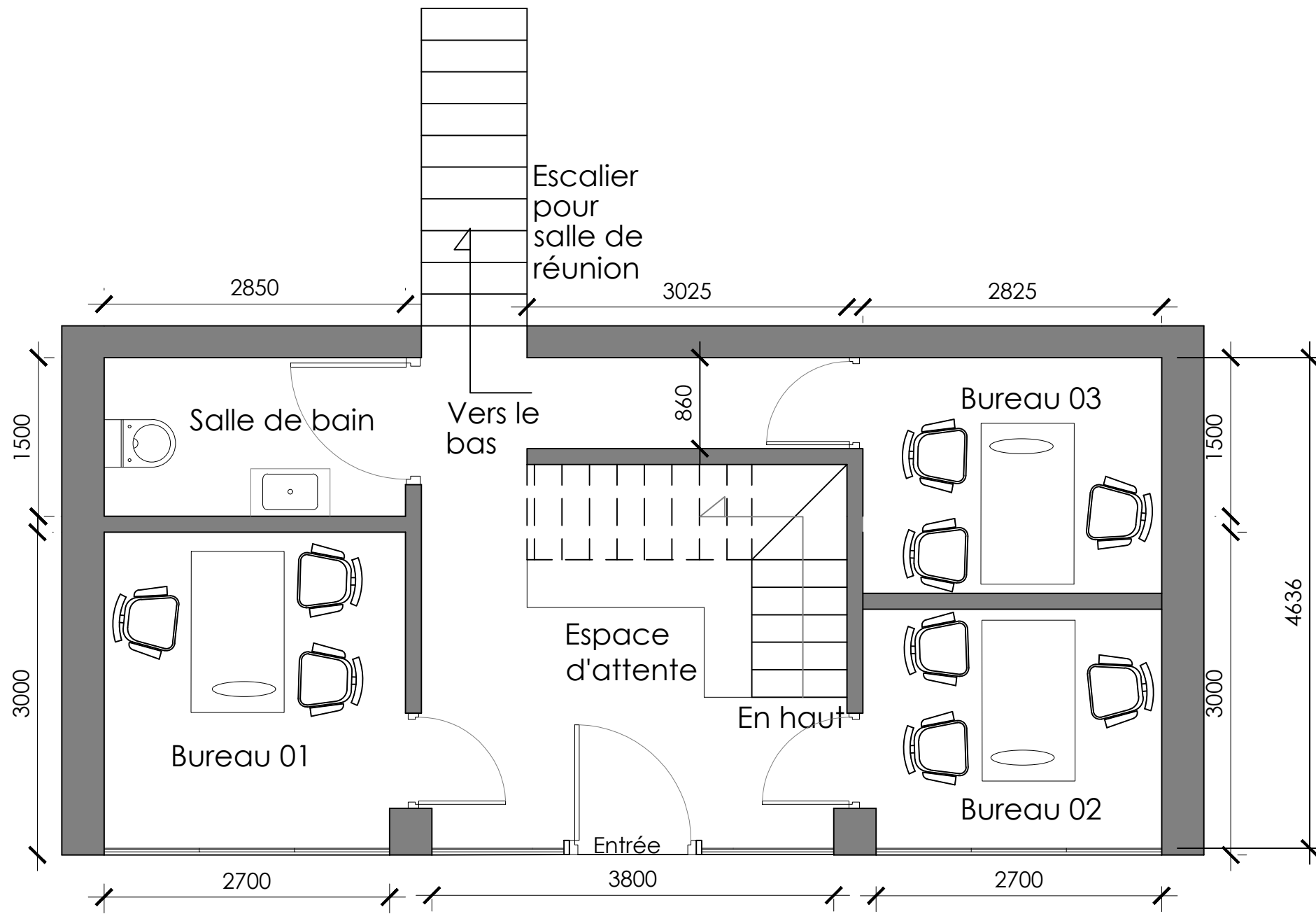
Plan du rez-de-chaussée Échelle 1:50
