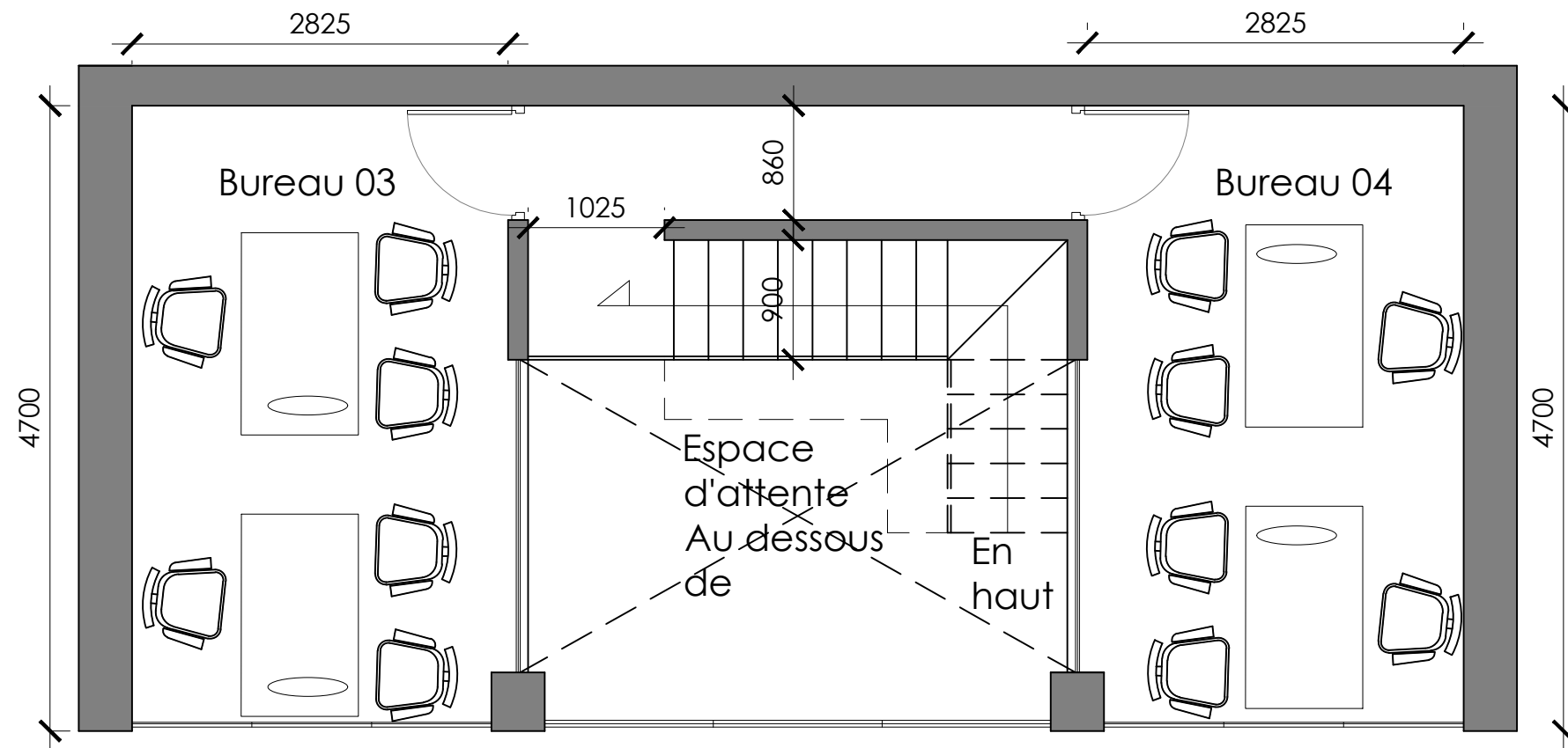
Plan du premier étage Échelle 1:50
